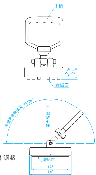
尺寸图 单位: mm
