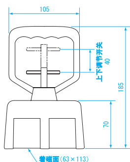
尺寸图 单位: mm
