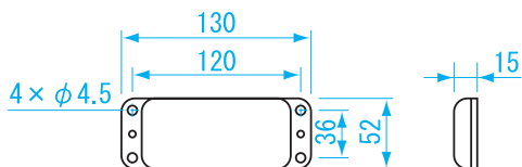
尺寸图 单位: mm
