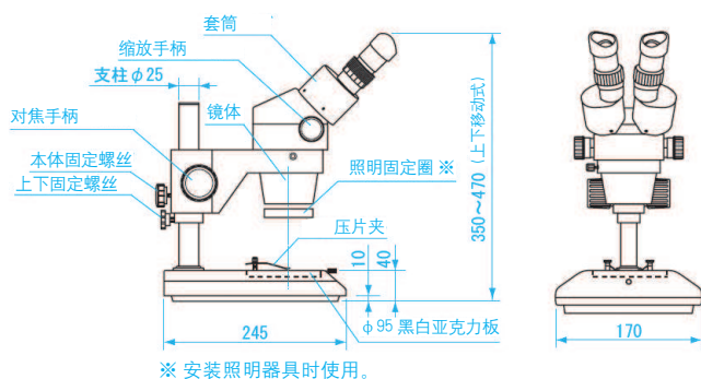
尺寸图
