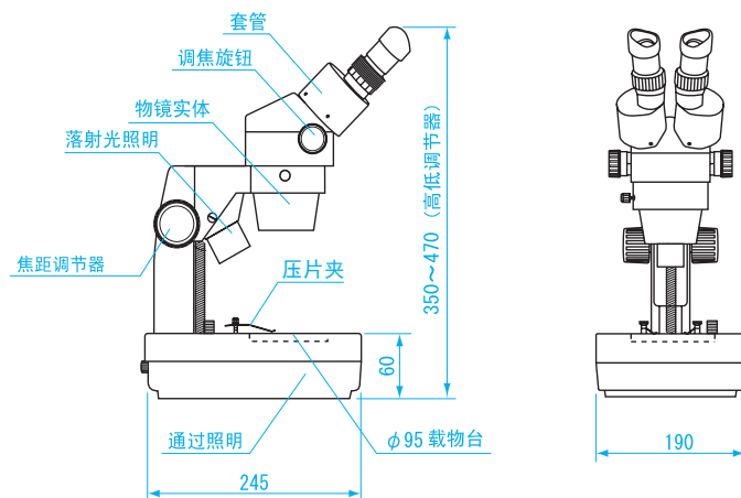
尺寸图
