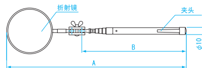
尺寸图 单位：mm
