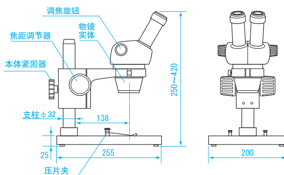
尺寸图
