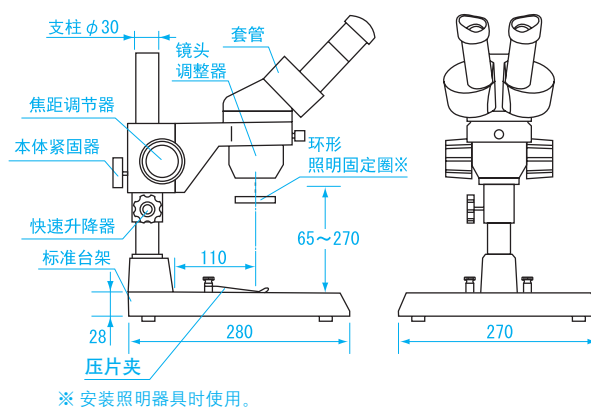
尺寸图
