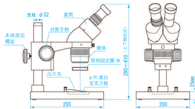
尺寸图
