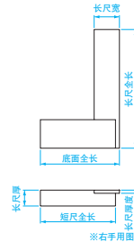
尺寸图
